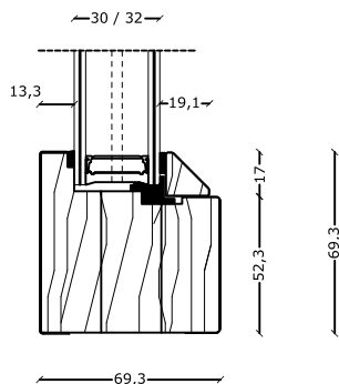
sezione verticale montante orizzontale fisso solo telaio
