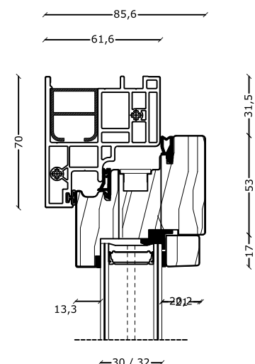
sezione verticale superiore anta in legno lamellare e telaio in pfv con con fermavetro minimal
