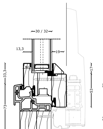
sezione soglia portafinestra
