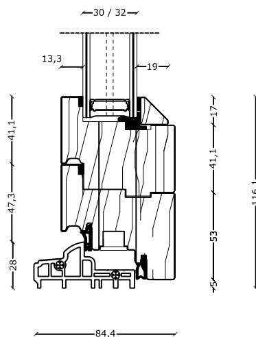
sezione soglia portafinestra
