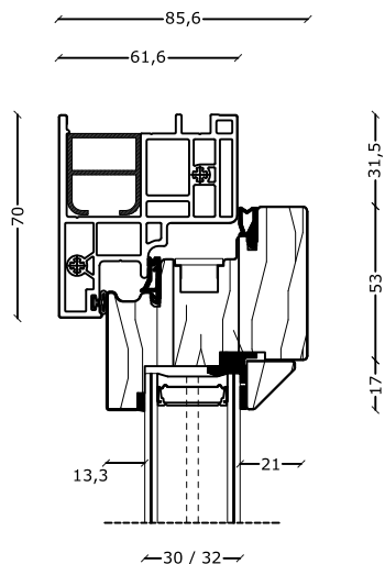
sezione verticale superiore anta in legno lamellare e telaio in pfv con con fermavetro design
