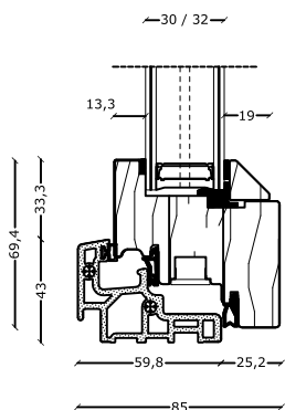
sezione gocciolatoio finestra
