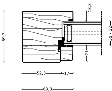
sezione orizzontale montante verticale fisso solo telaio
